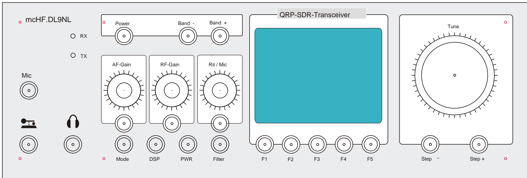
Frontplattenentwurf DL9NL
